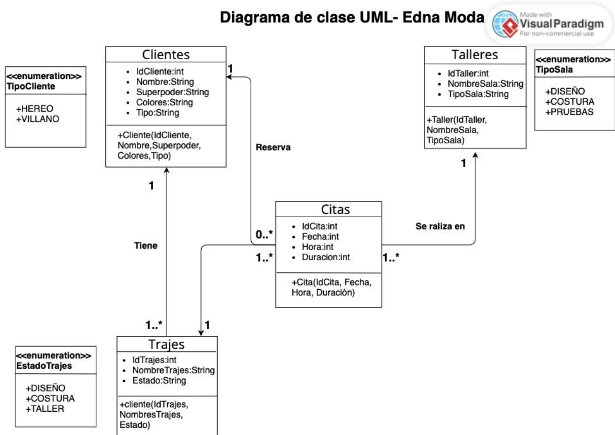
Figura 9. Diagrama de Clase
